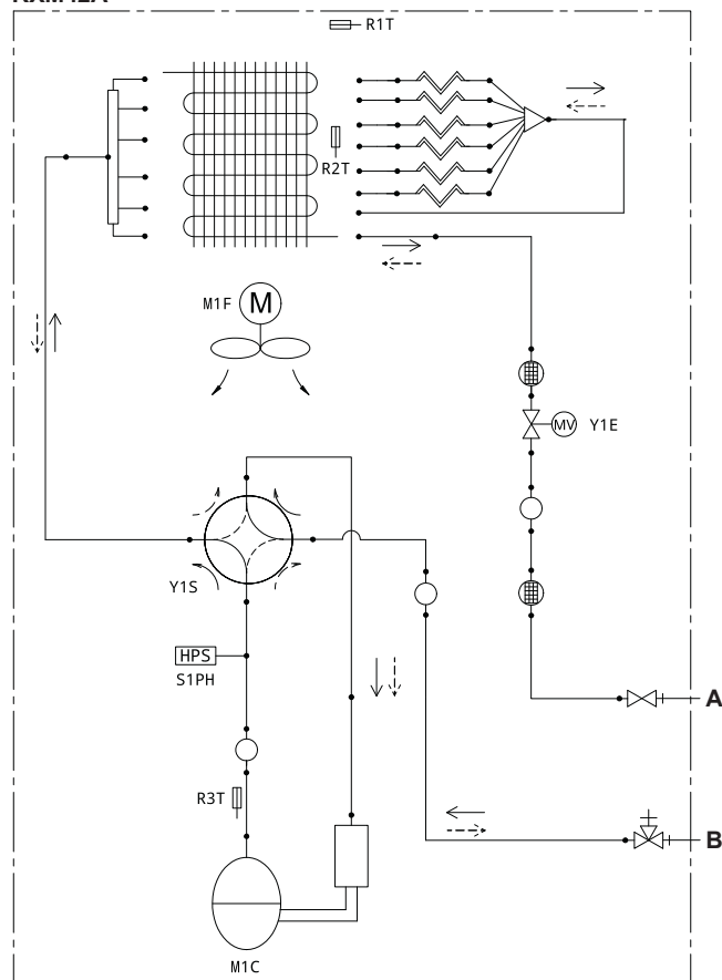
Schema delle tubazioni
